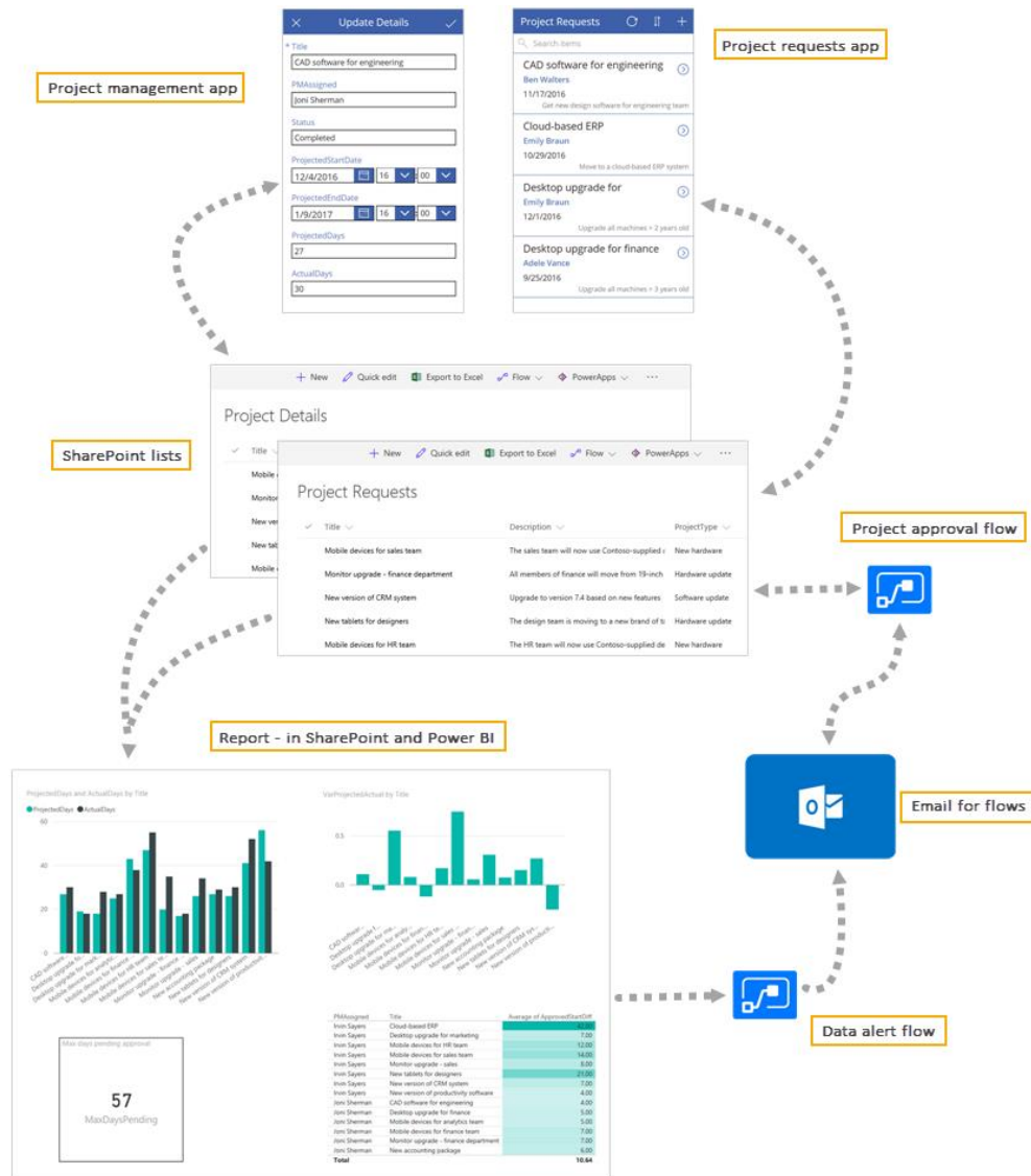
Figura 2 – Modelo estrutural descreve integração pelos conectores - aplicativo tela Power apps, obtenção de dados em nuvem pelo Sharepoint, uso disparo automatizado de email com Power Automate e geração de interface gráfica (dashboards) Power BI (MICROSOFT, 2023).
